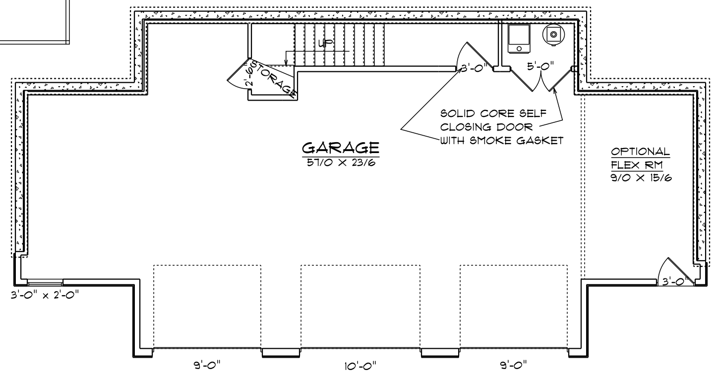
BASEMENT LAYOUT SCALE: 1/8" = 1'-0"
